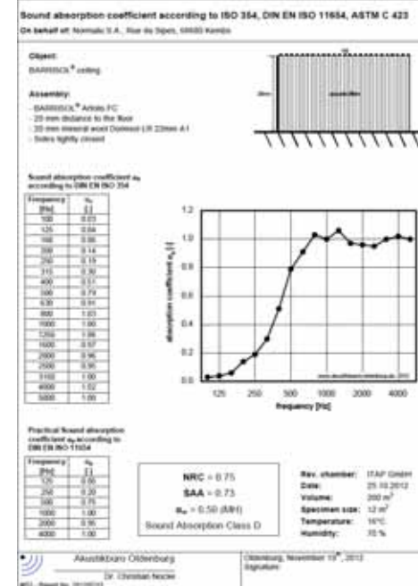
artolis acoustic® + 20 mm laine de verre
